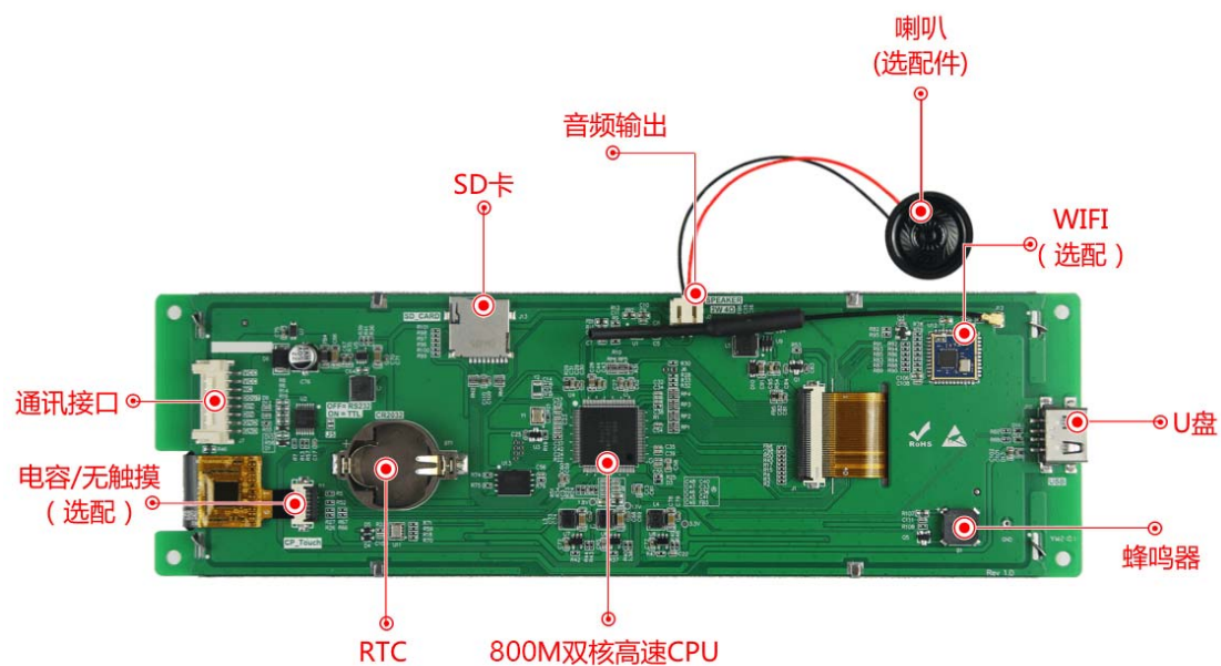
图 1-3 硬件配置图
