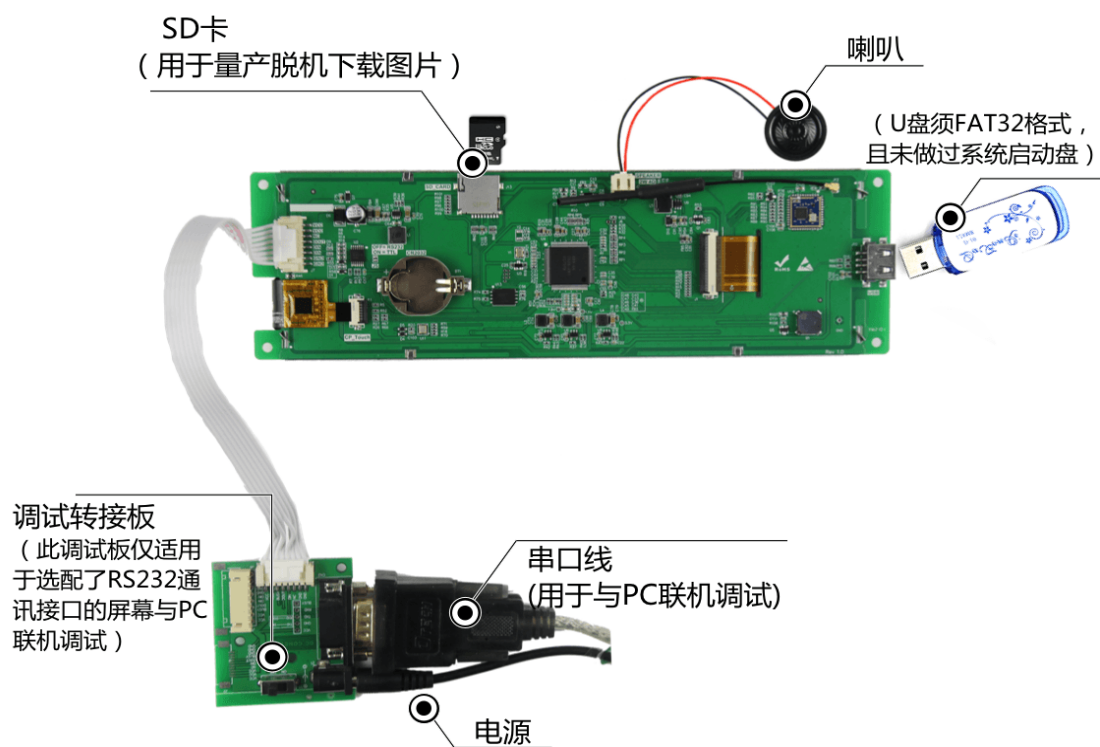
图 1-4 调试工具
